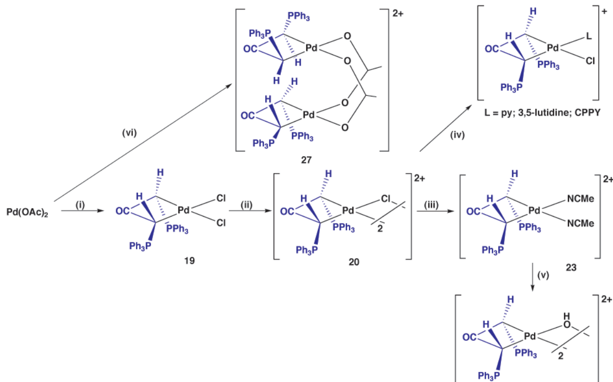
Scheme 3 (i) + [\text{Ph}_3\text{PCH}_2\text{COCH}_2\text{PPh}_3]\text{Cl}_2 , -2 \text{HOAc} , \text{CH}_2\text{Cl}_2 , r.t. (ii) + \text{TiClO}_4 , -\text{TiCl} , \text{CH}_2\text{Cl}_2 , r.t. (iii) + 2 \text{TiClO}_4 , -2 \text{TiCl} , \text{NCMe} , r.t. (iv) + 2 \text{L} , \text{CH}_2\text{Cl}_2 , r.t. (v) + 2 \text{NBu}_4\text{OH} , \text{MeOH}/\text{H}_2\text{O} , r.t. (vi) + [\text{Ph}_3\text{P}=\text{C}(\text{H})\text{COCH}_2\text{PPh}_3](\text{ClO}_4) , -\text{HOAc} , \text{CH}_2\text{Cl}_2 , r.t.
